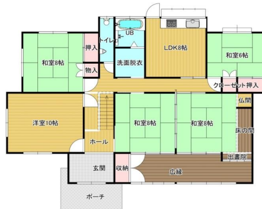
1F平面図
