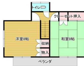
2F平面図
